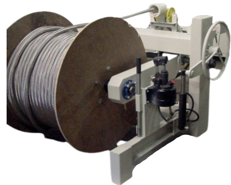
UNWINDER DE TOURET
